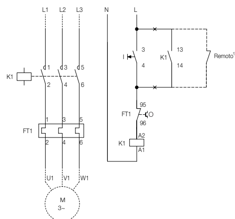
Figura 2 (alimentación del circuito de mando separada de la red)
