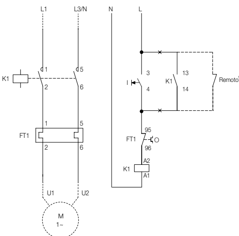
Figura 2 (alimentación del circuito de mando separada de la red)
